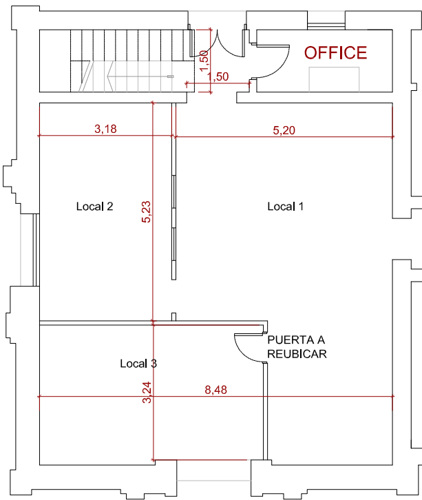
PLANTA ACTUAL
