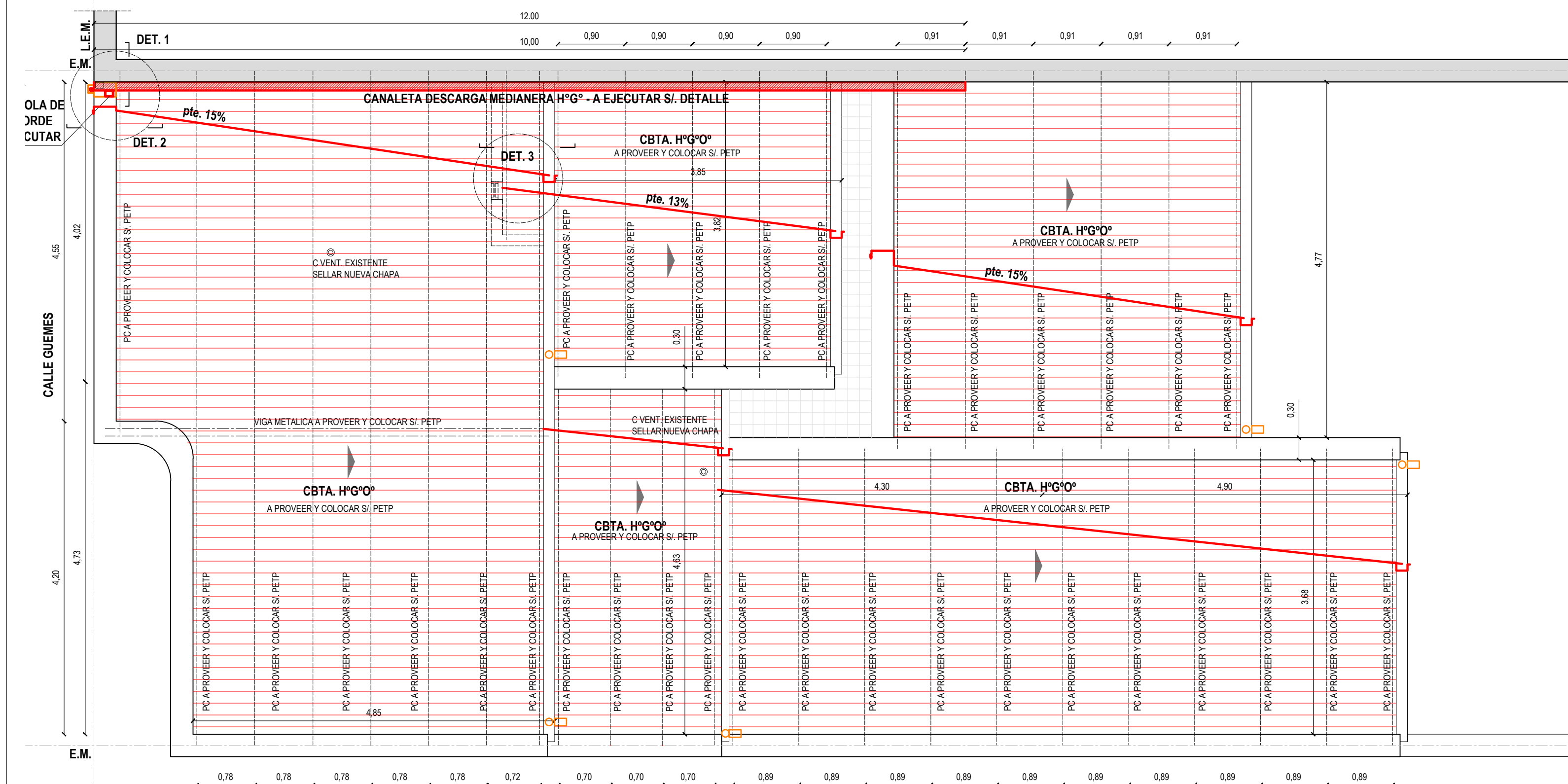
PLANTA DE TECHOS - SECTOR A INTERVENIR TRABAJOS A EJECUTAR
