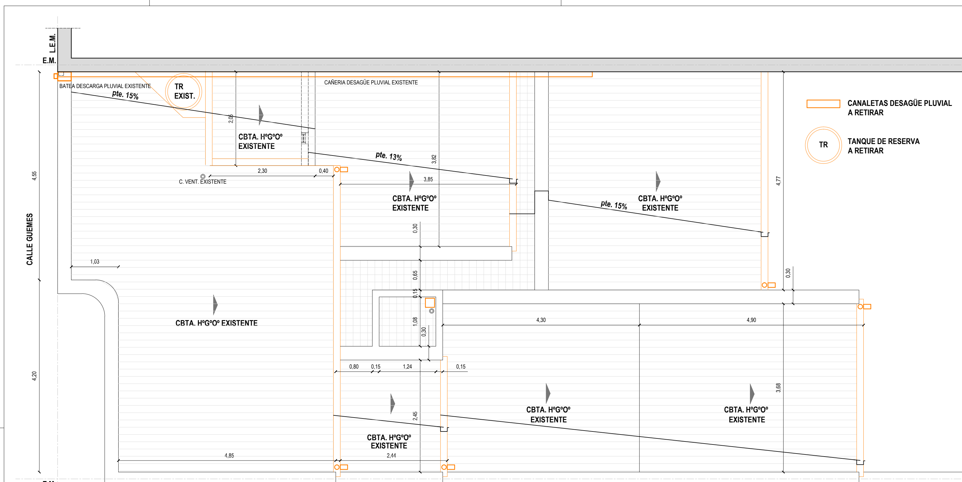
PLANTA DE TECHOS - SECTOR A INTERVENIR SITUACION ACTUAL
