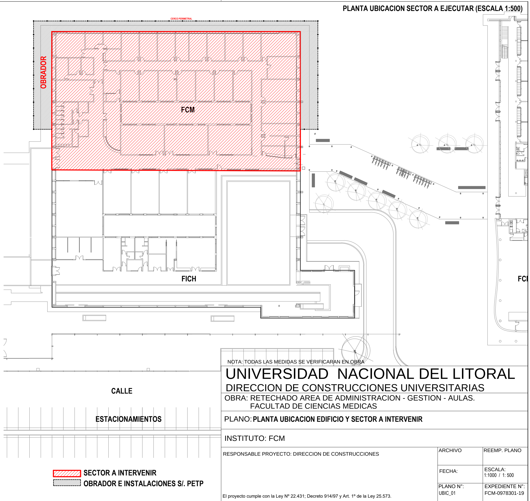
PLANTA UBICACION SECTOR A EJECUTAR (ESCALA 1:500)
