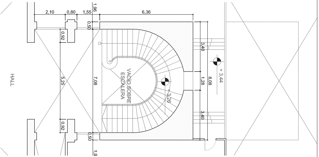
PLANTA ENTREPISOS ESC. 1:100
