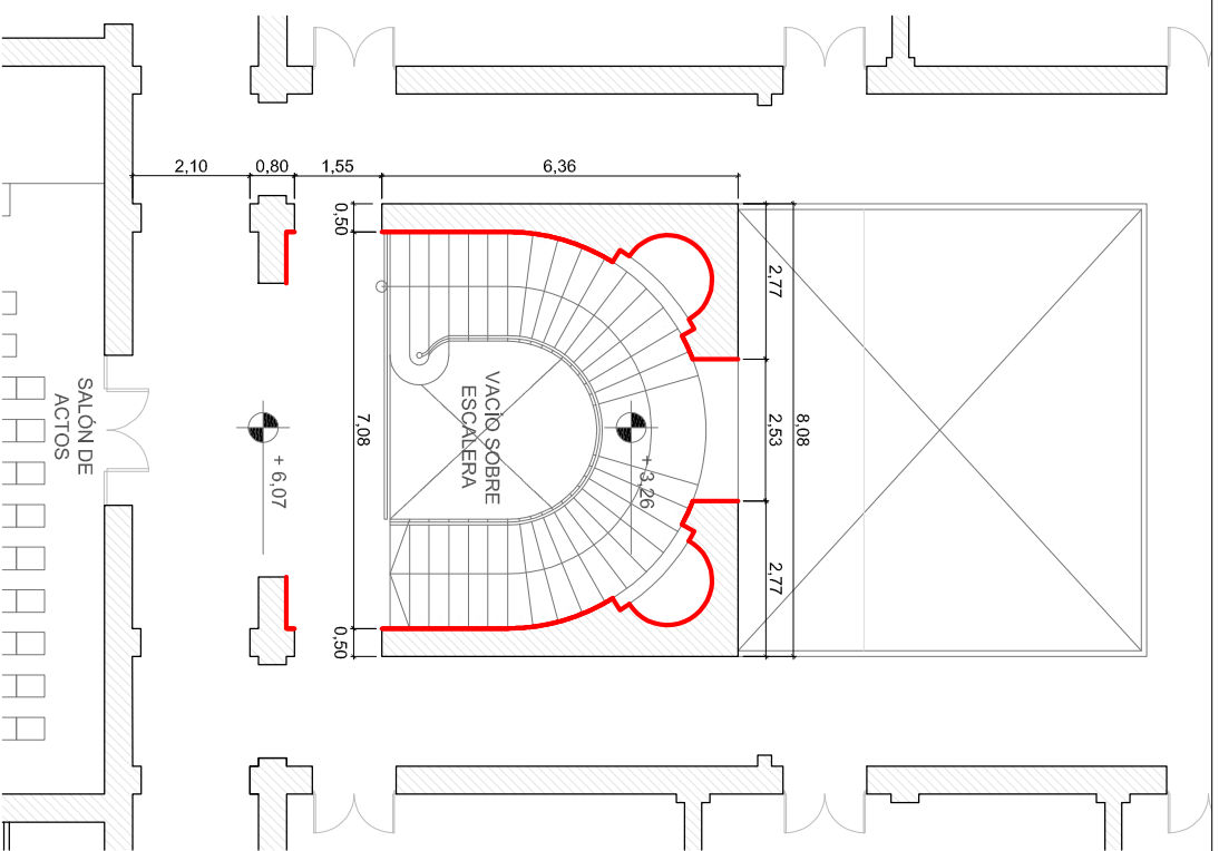
PRIMER PISO ESC. 1:100
