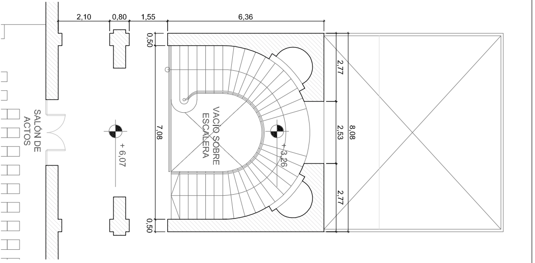
PRIMER PISO ESC. 1:100
