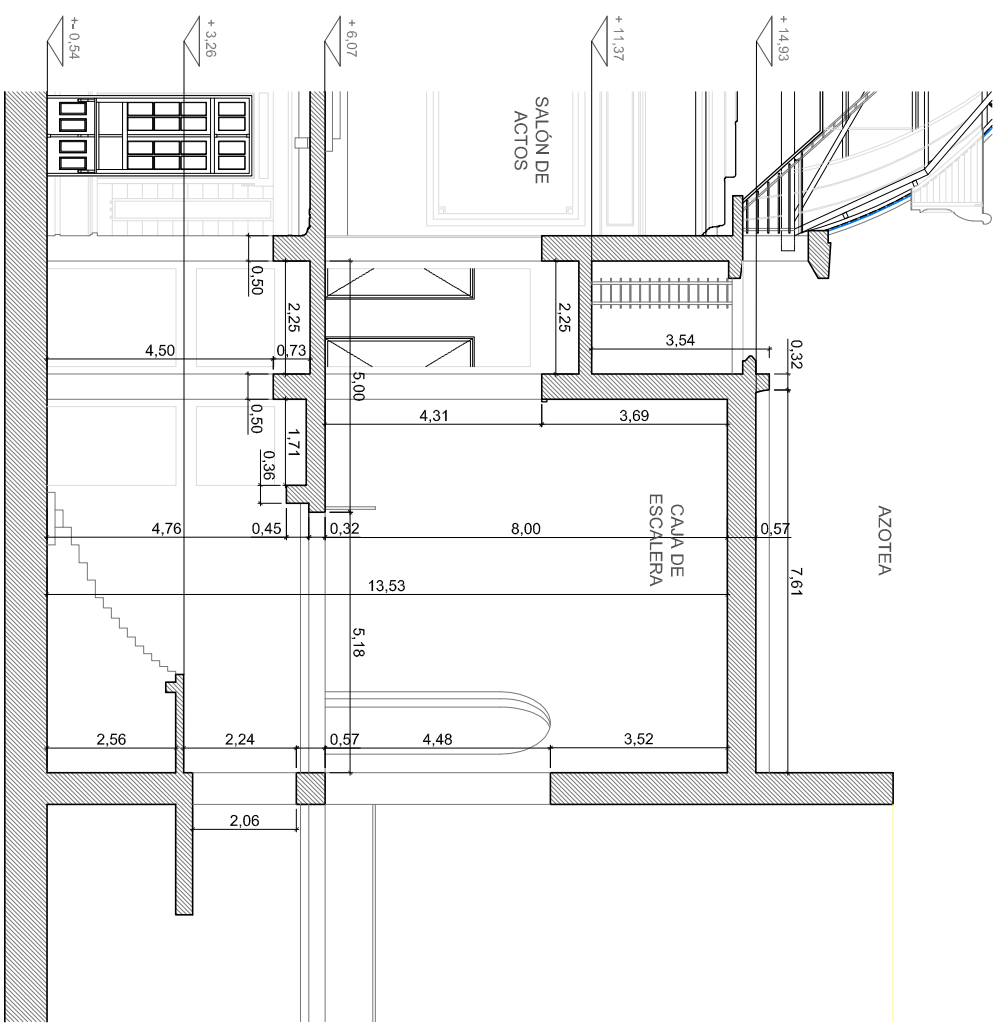
CORTE LONGITUDINAL ESC. 1:100
