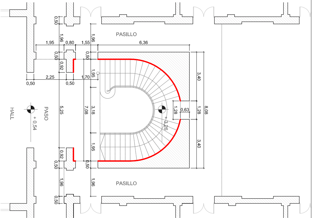
PLANTA BAJA ESC. 1:100
