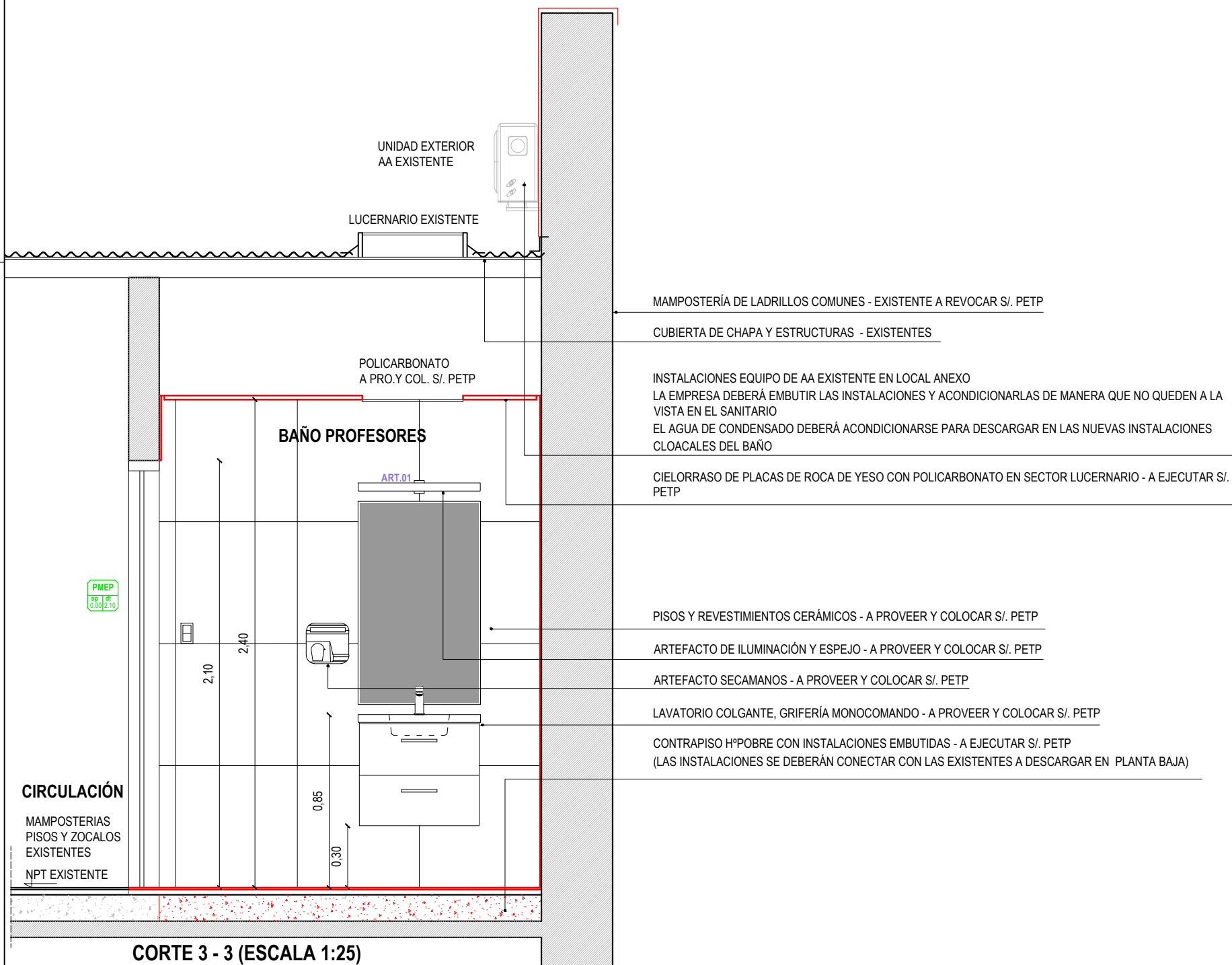
CORTE 3 - 3 (ESCALA 1:25)
