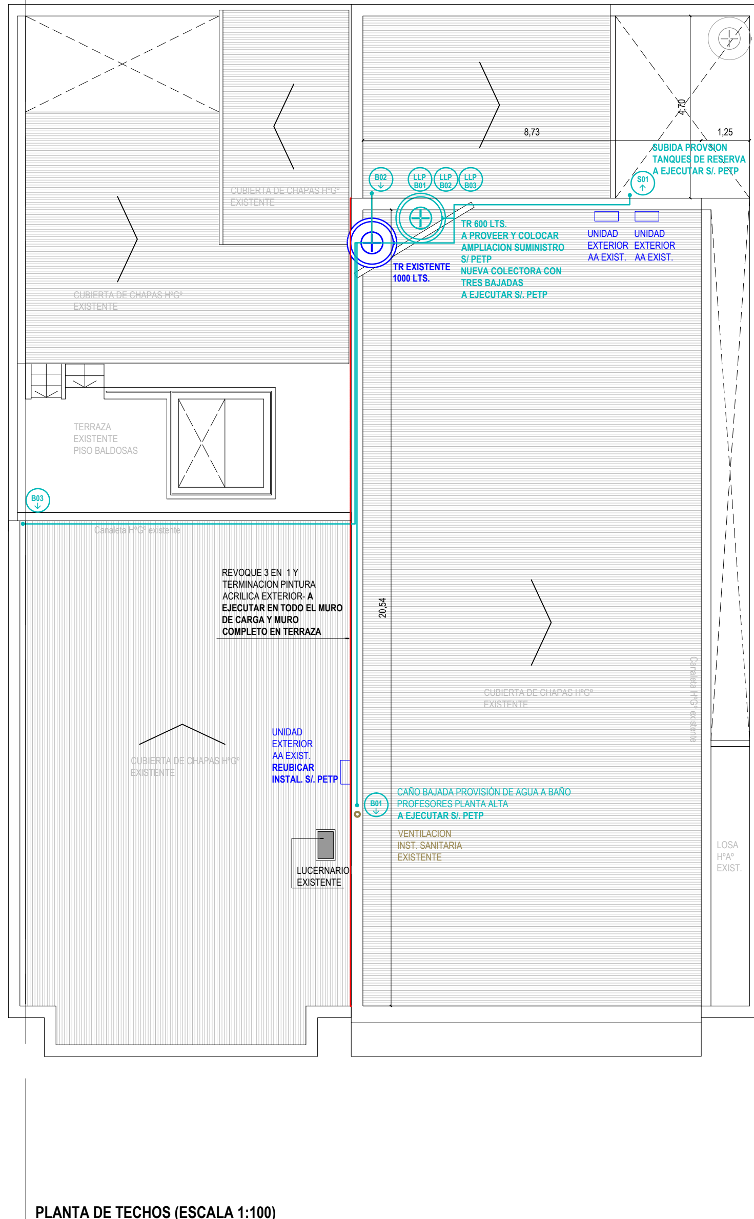
PLANTA DE TECHOS (ESCALA 1:100)
