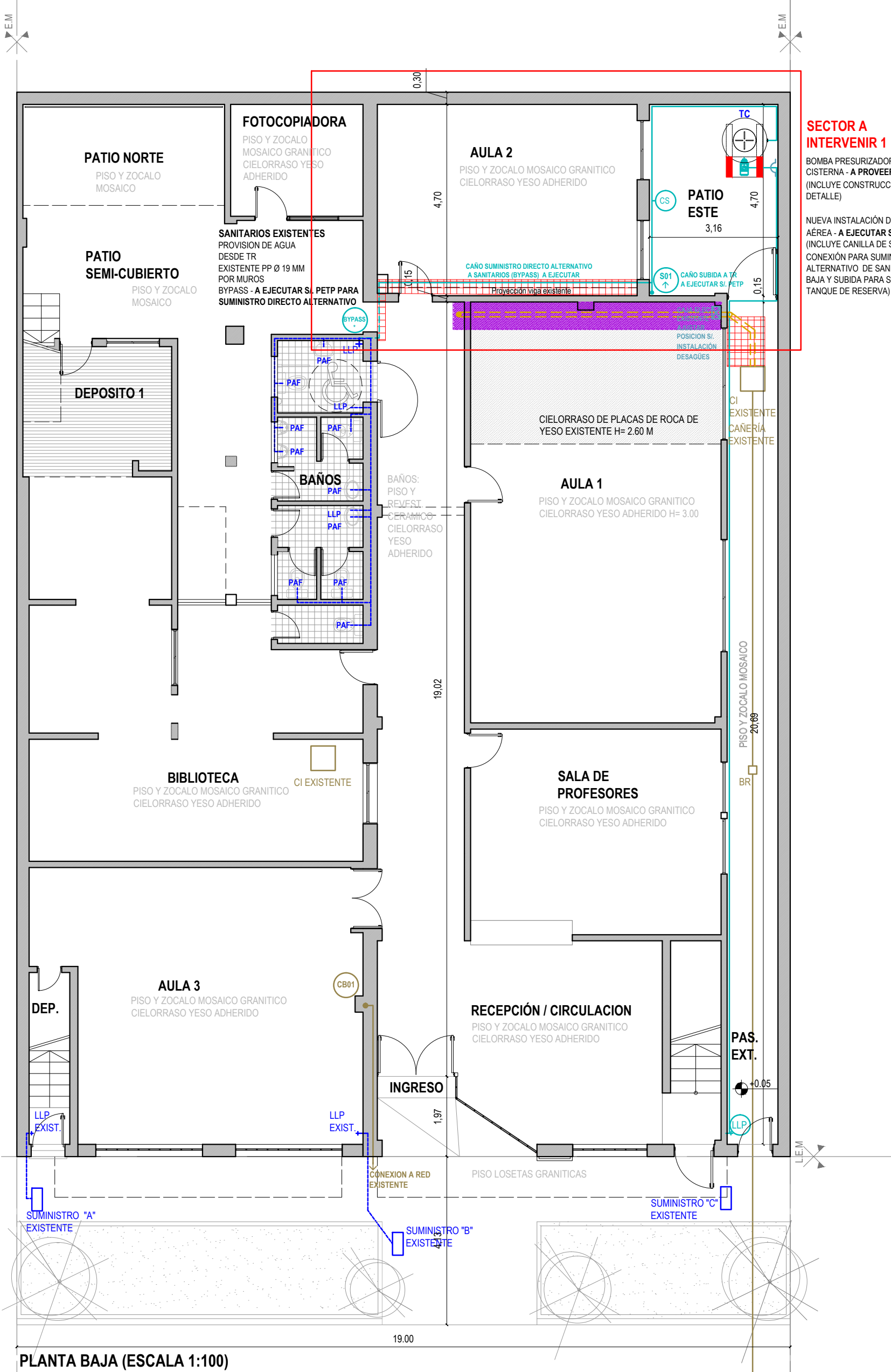
PLANTA BAJA (ESCALA 1:100)
