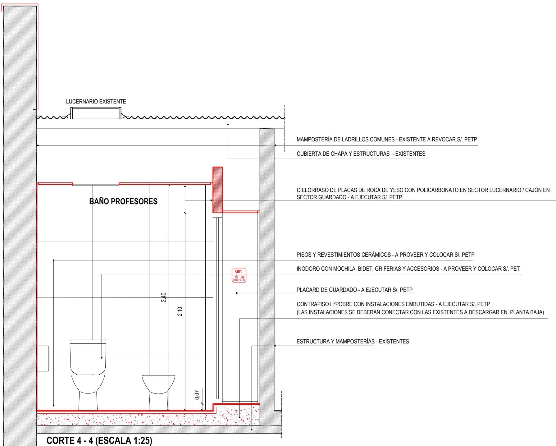
CORTE 4 - 4 (ESCALA 1:25)
