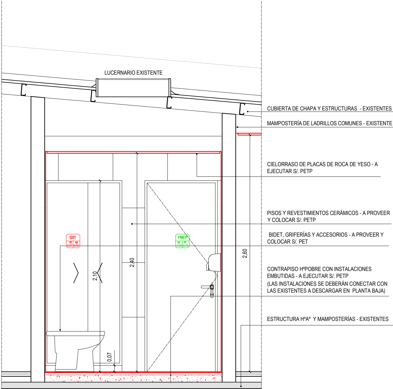
CORTE 1 - 1 (ESCALA 1:25)
