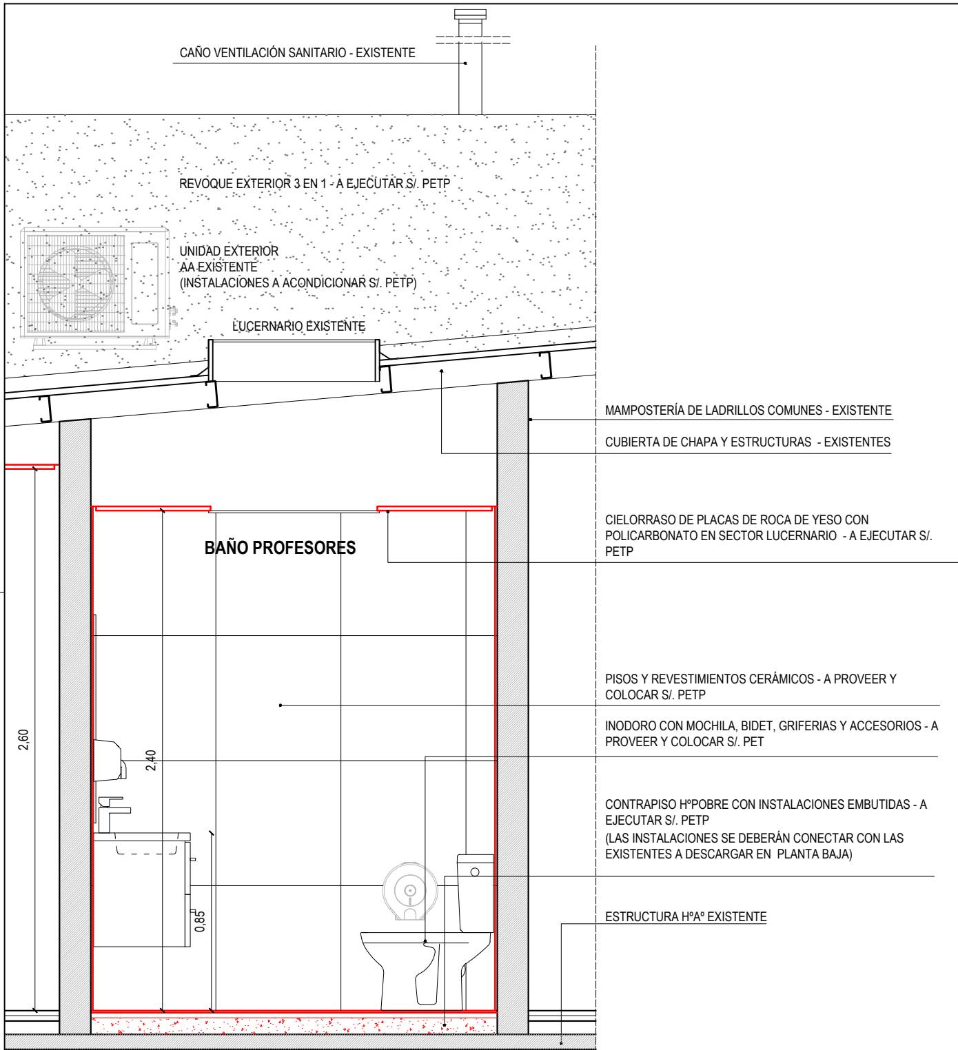
CORTE 2 - 2 (ESCALA 1:25)
