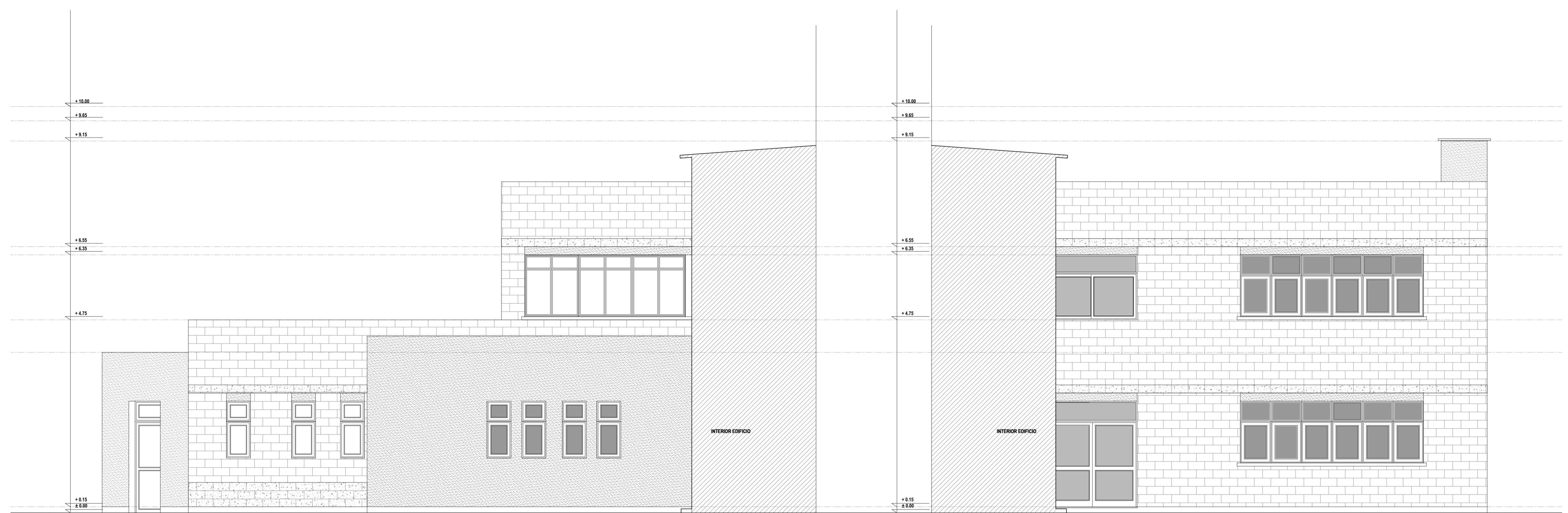
CORTE 1 - 1 (VISTA ESTE PATIO)
